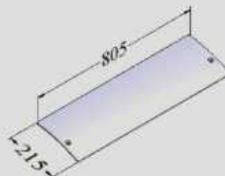
CARENAGEM FRONTAL SEM RASGO COD - VC0020
