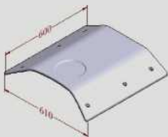
CARENAGEM SUPERIOR GRANDE TRASEIRA SEM RASGO COD - VC00230
