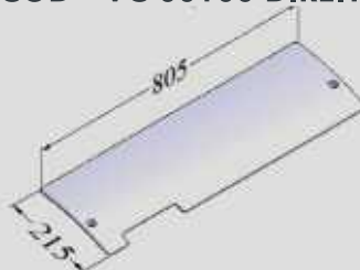
CARENAGEM INFERIOR FRONTAL COM RASGO COD - VC 00100 DIREITA
